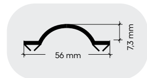
Perfil / Section
